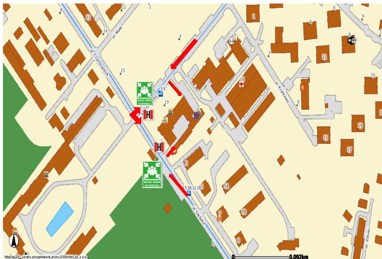
Rysunek. Układ dróg dojazdowych oraz rozmieszczenie hydrantów przeciwpożarowych.
