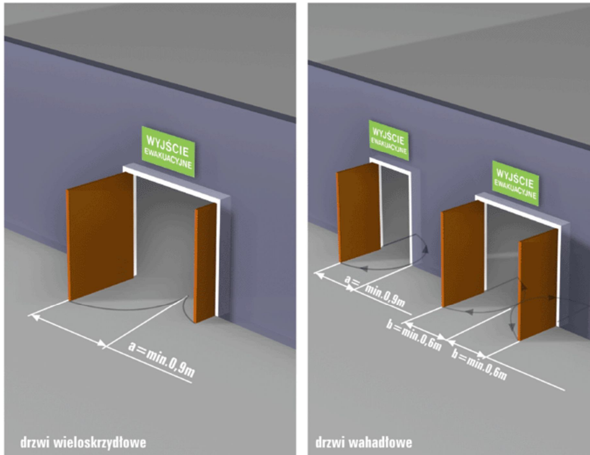
Rysunek. Zasada określania parametrów wyjść ewakuacyjnych .
