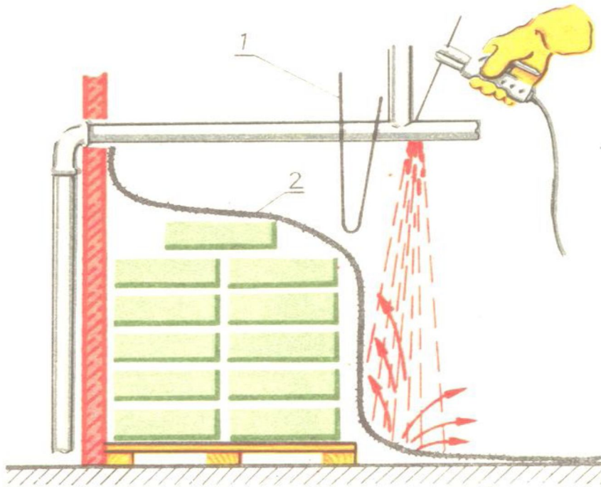
Rysunek.1. Palne materiały, których usunięcie poza zasięg rozprysków spawalniczych jest niemożliwe, osłaniamy w sposób gwarantujący bezpieczeństwo: 1-ekran z blachy, 2-koc gaśniczy.
