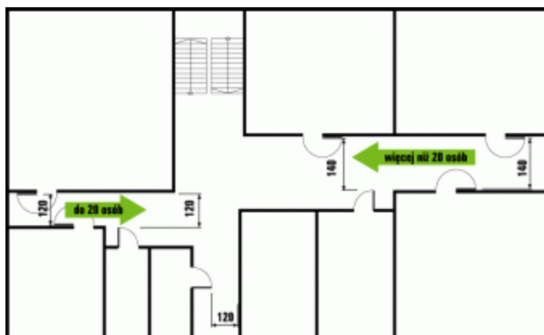
Rysunek. Zasady określania dość ewakuacyjnych.
