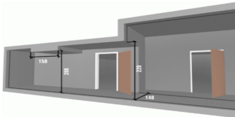
Rysunek. Parametry poziomych dróg ewakuacyjnych.
