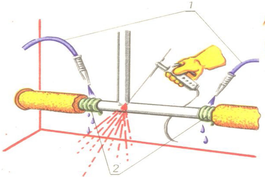
Rysunek. 4. Z izolowanych rurociągów, na których prowadzi się prace spawalnicze, należy usunąć izolację cieplną na odcinku gwarantującym bezpieczeństwo, a w razie potrzeby (izolacja łatwopalna) chłodzić skutecznie np. sposobem pokazanym na rysunku: 1-przewody doprowadzające wodę, 2-zwoje sznura z włókna niepalnego.
