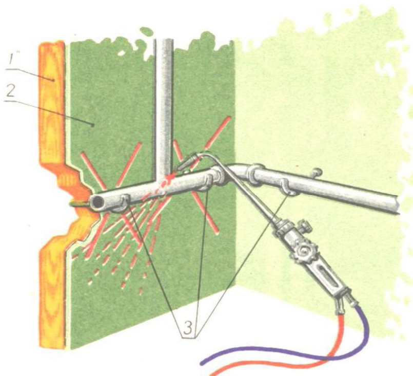
Rysunek. 5. Elementy instalacji rozgrzewające się przy spawaniu bezpośrednio od płomienia lub na drodze przewodnictwa cieplnego, stykające się z materiałami palnymi, należy zdemontować lub skutecznie chłodzić: 1-palna ścianka, 2-niepalna wykładzina, 3-haki podtrzymujące instalację.
