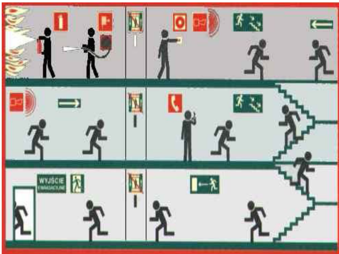
Rysunek .Sposób rozmieszczania znaków ewakuacyjnych i bezpieczeństwa.
