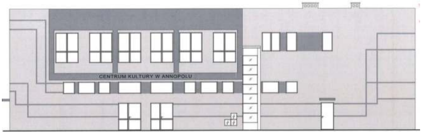
ELEWACJA PÓLNOČNA
