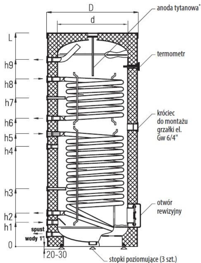
Wymiennik SGW(S)B 300-500 l
