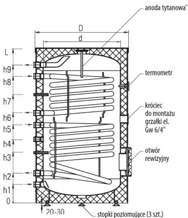
Wymiennik SGW(S)B 200 l
