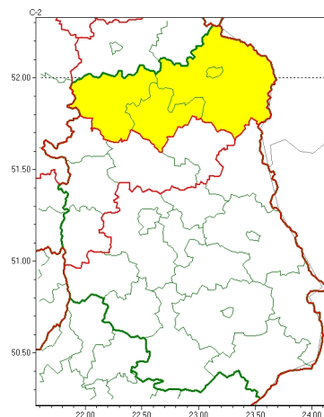
Zawieje/zamiecie śnieżne 2022-12-10 23:45
