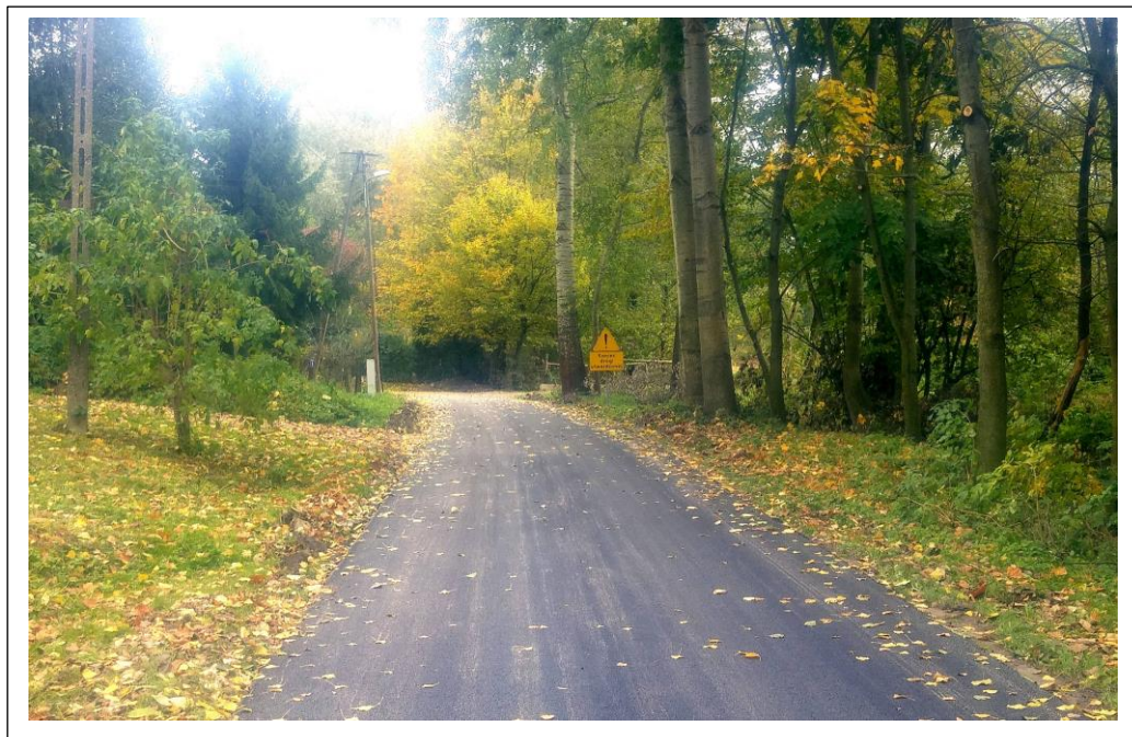
Fot. 13. Przebudowany odcinek drogi wewnętrznej w miejscowości Łubki na długości 100 m.
